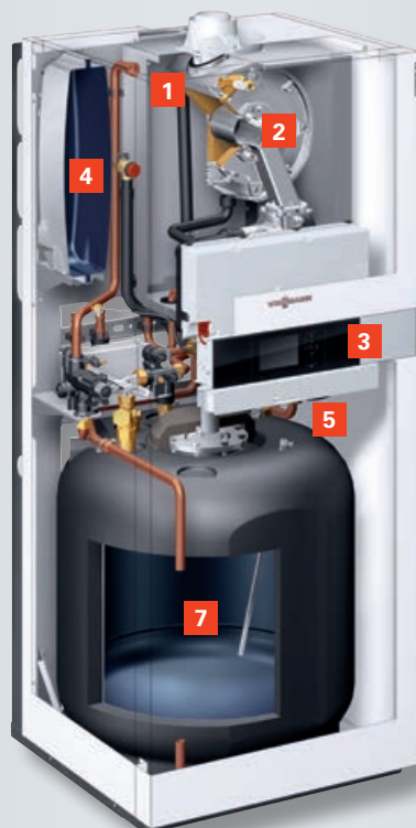
Vitodens 222-F (type B2TB) avec ballon en acier émaillé à système de charge
